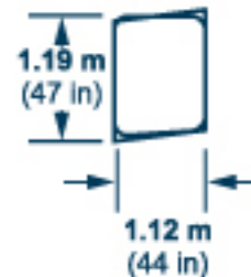
Bulk cargo door (STA 2007) Right-hand side
