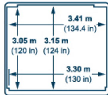
Main deck cargo door (STA 1770) Left-hand side
