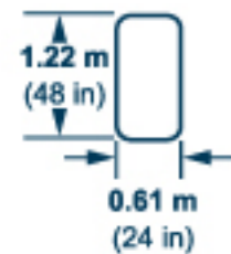
U/D entry door (STA 464) Left-hand side
